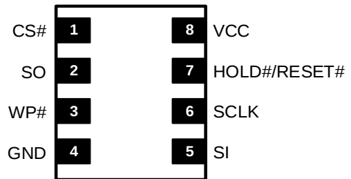
8-Pad USON(3x2mm/1.5x1.5mm)
